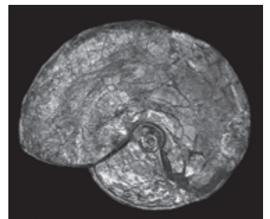
▲アンモライト
