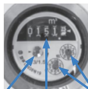
パイロット カウンター(m) 赤い針(ℓ)
